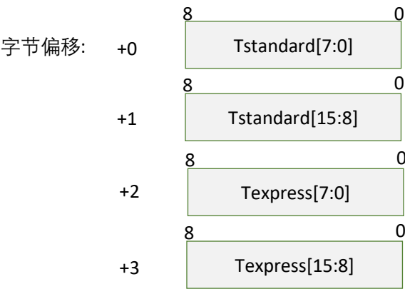
图表 4-23 激光测距用时获取请求对应的数据应答报文
