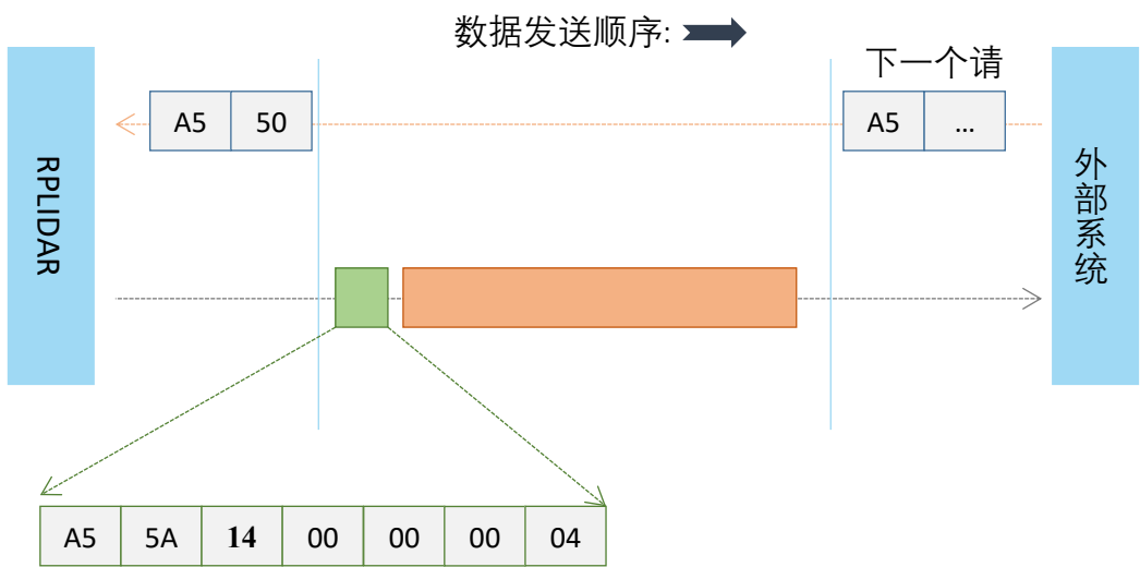
图表 4-20 GET_INFO 请求的通讯时序
