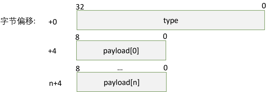
图表 4-27 设备配置信息获取命令请求对应的数据应答报文
