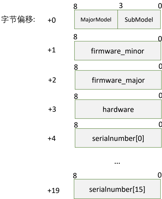
图表 4-18 设备信息获取对应的数据应答报文
