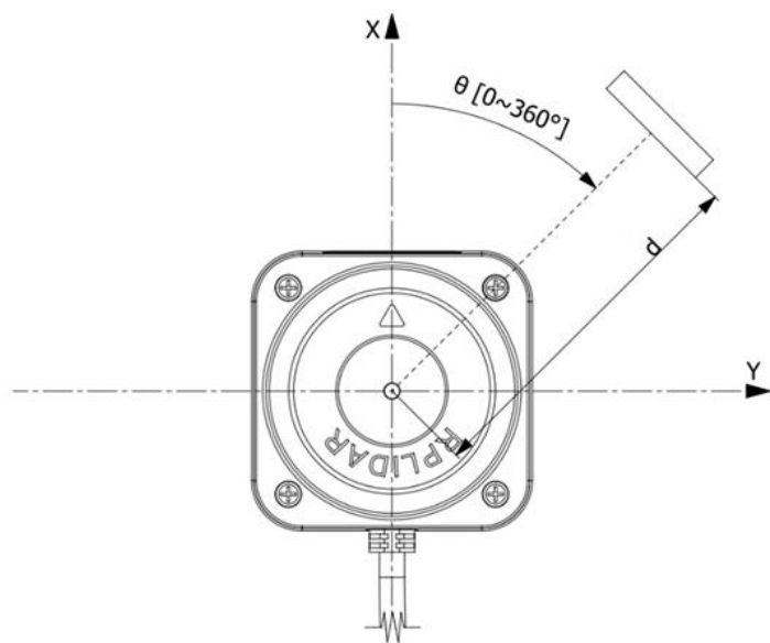
图表 4-9 RPLIDAR C1 测距时夹角与距离值几何定义
