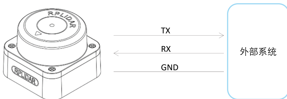
图表 1-1 RPLIDAR 与外部系统通讯示意图
