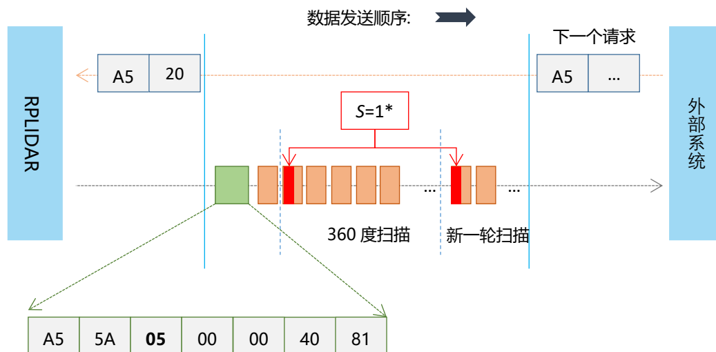
图表 4-10 外部系统发送扫描采样请求后的通讯情况
