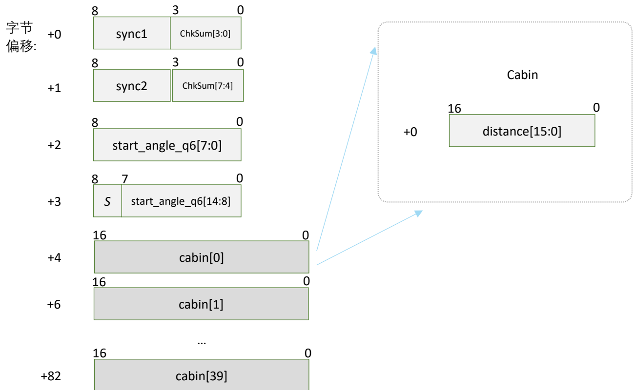
图表 4-13 高速扫描测距输出的数据应答报文格式
