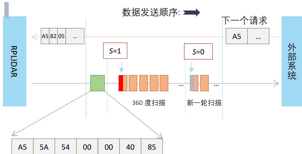
图表 4-16 外部系统在发送高速采样请求后的通讯情况
