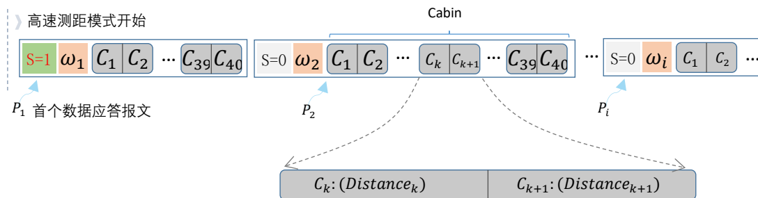
图表 4-17 高速测距模式（密实模式）中发送出的应答报文抽象表示
