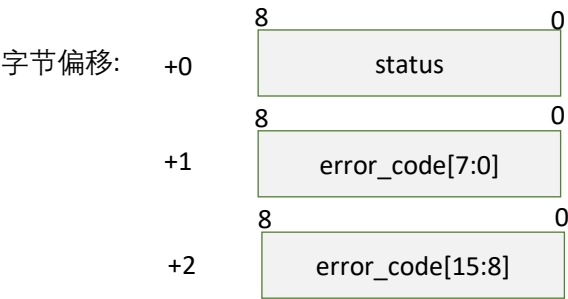
图表 4-21 设备健康状态请求对应的数据应答报文
