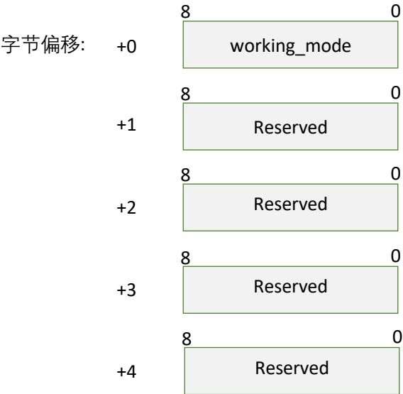
图表 4-11 高速采样模式请求报文的数据格式
